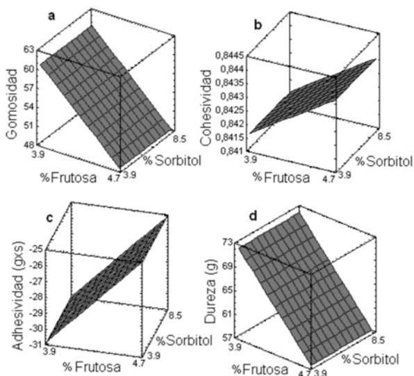
Figura 4. Superficie de respuesta (textura), prueba instrumental
